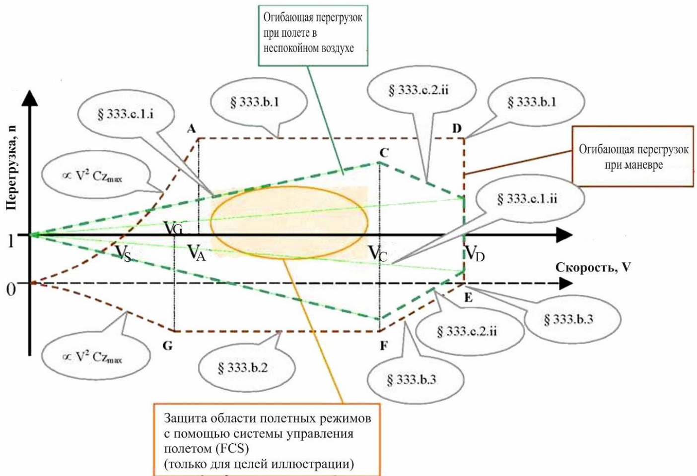
Рисунок С1. Область полетных режимов
